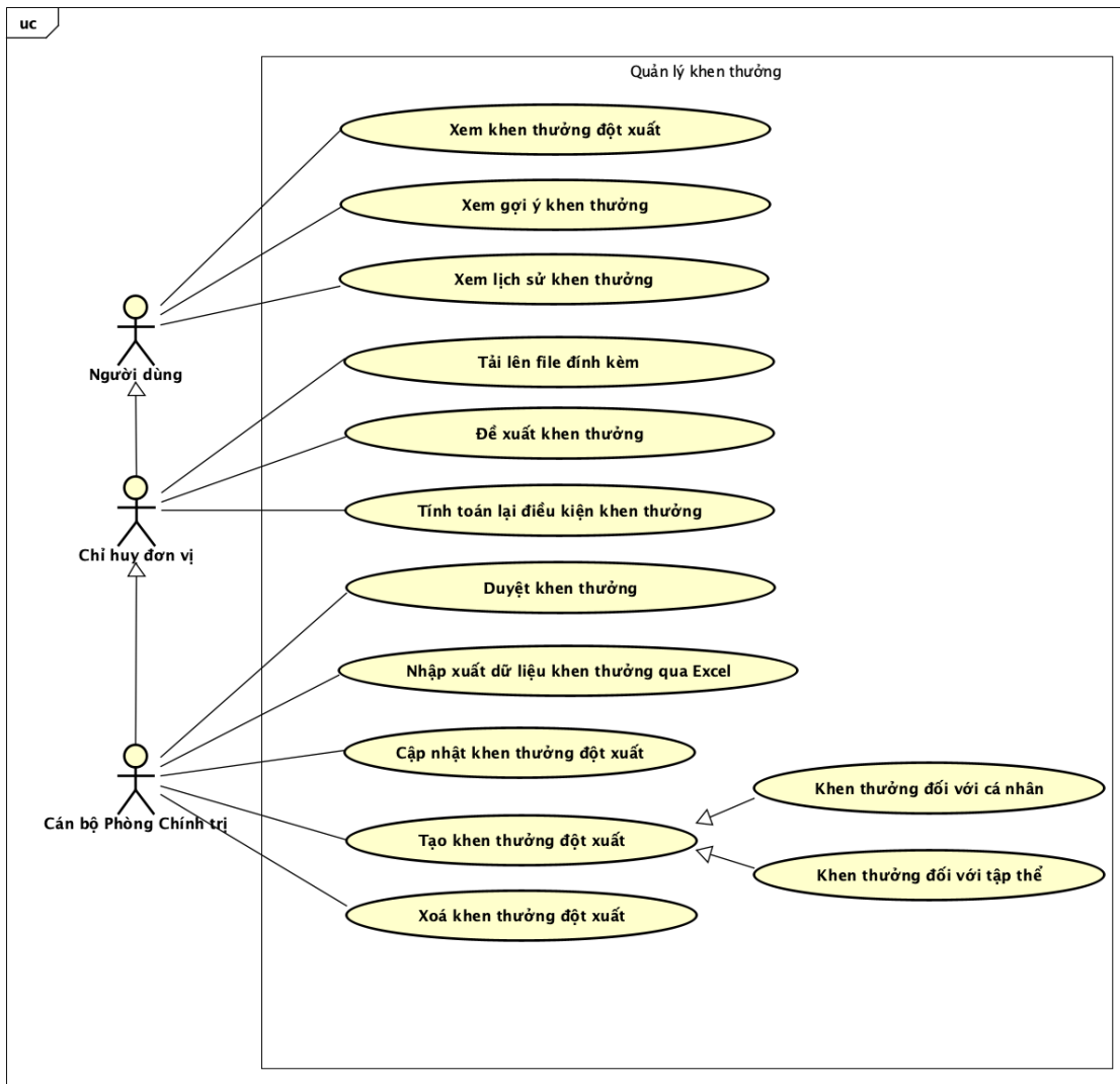
Hình 0.4: Biểu đồ use case phân rã chức năng quản lý khen thưởng
