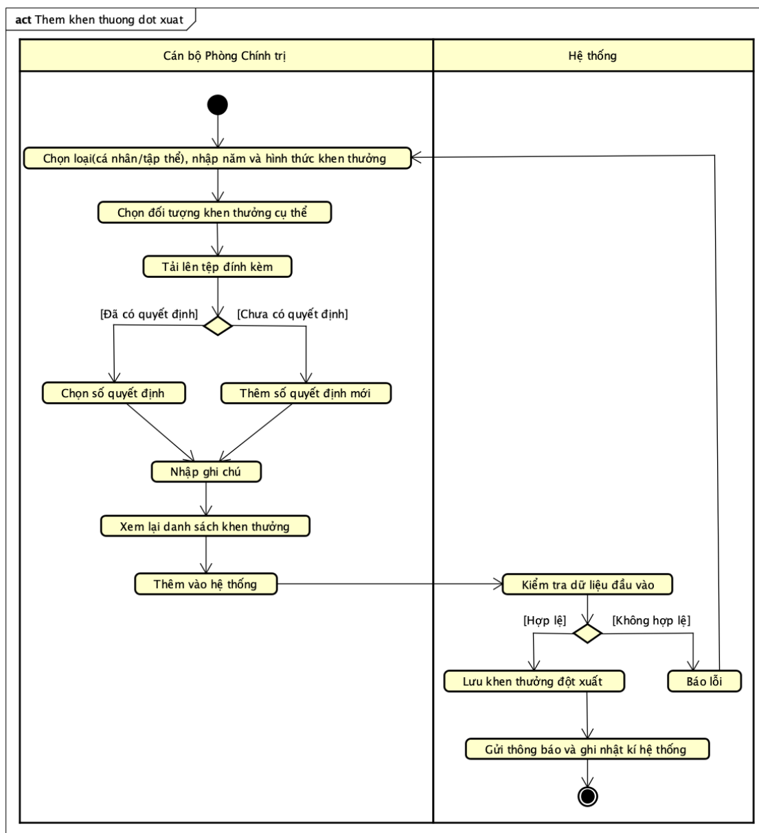
Hình 0.10: Biểu đồ hoạt động quy trình thêm khen thưởng đột xuất
