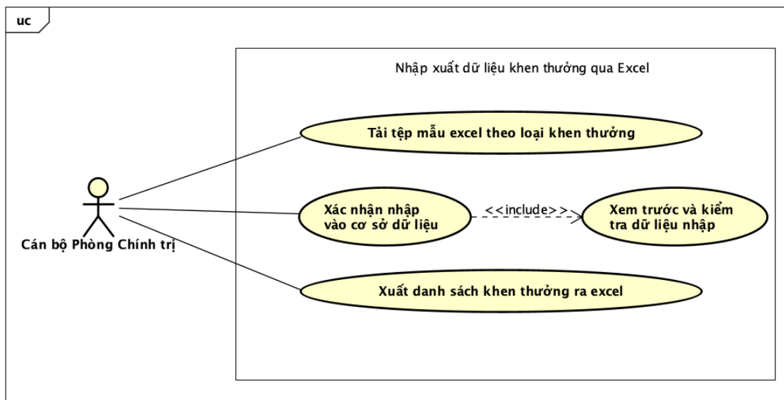
Hình 0.5: Biểu đồ use case phân rã chức năng nhập và xuất dữ liệu Excel
