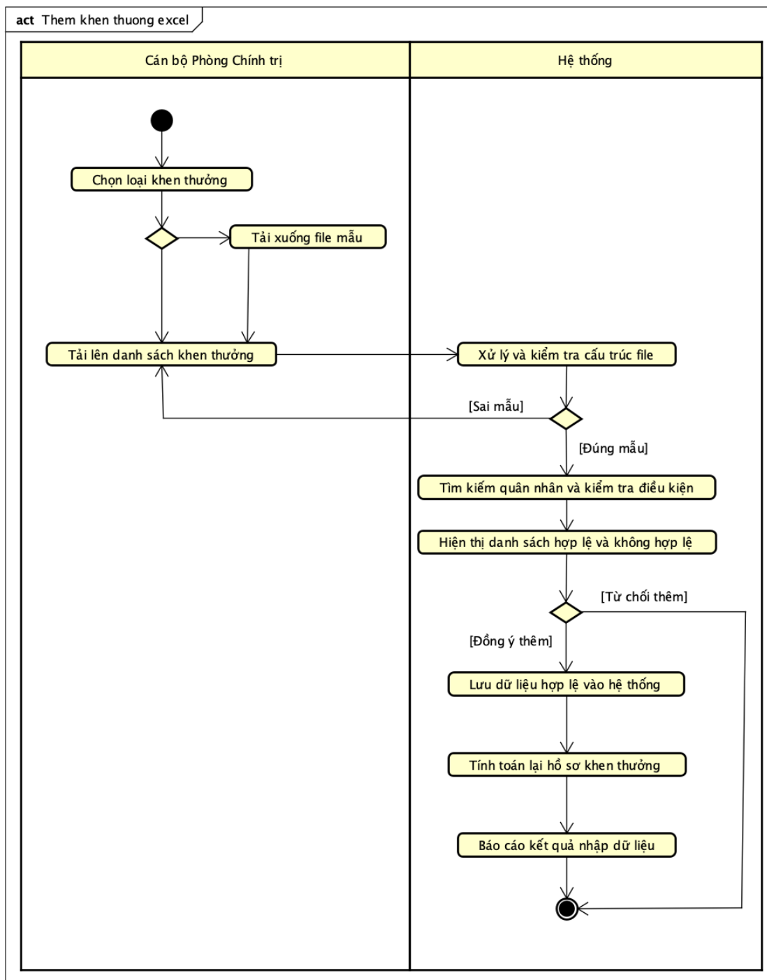
Hình 0.9: Biểu đồ hoạt động quy trình nhập khen thưởng từ tệp Excel
