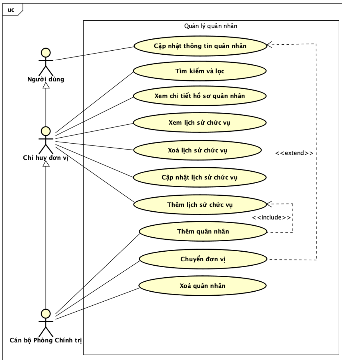
Hình 0.2: Biểu đồ use case phân rã chức năng quản lý quân nhân
